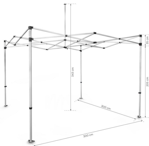
Gestellmaße: 300 x 300 cm, Durchgangshöhe 205 cm, Gesamthöhe 343 cm
