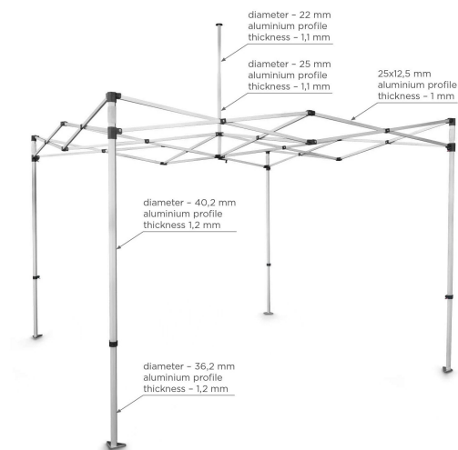
Aluminiumprofile: Beine 40,2 / 36,2 mm, Dachstreben 25 x 12,5 mm, Mast 25 / 22 mm
